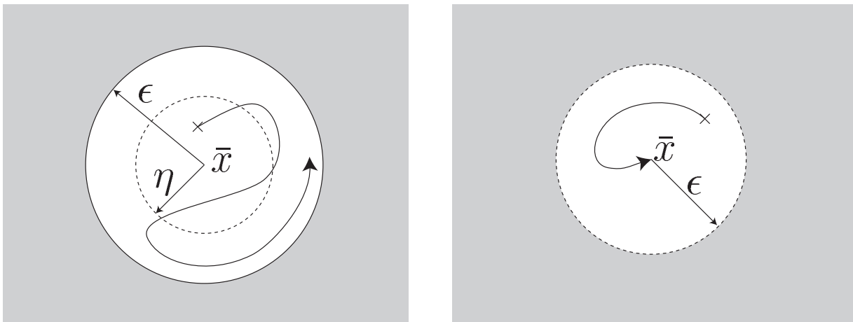
FIGURE 1.3 – Stabilité (gauche) et stabilité asymptotique (droite).
