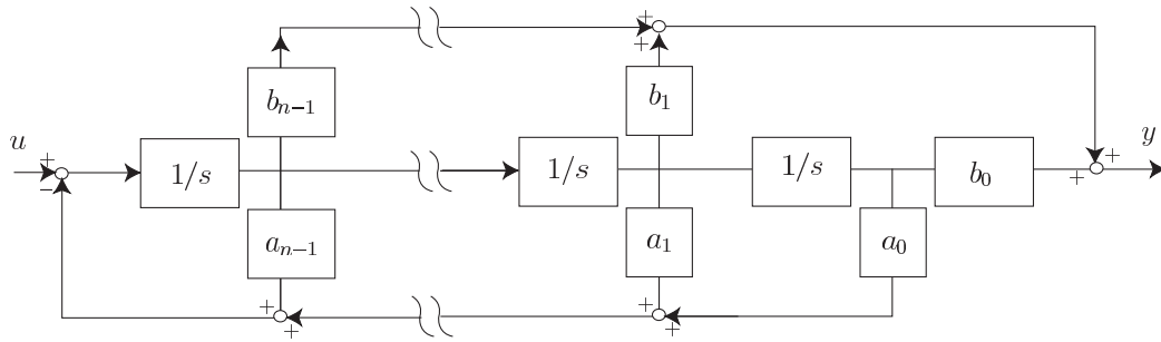
FIGURE 2.1 – Réalisation d'une fonction de transfert strictement propre.
