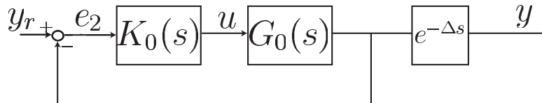
FIGURE 2.20 – Forme équivalente du système bouclé avec prédictiveur de Smith.
