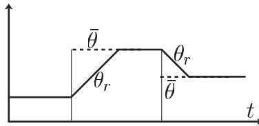
FIGURE 1.22 – Approximation de la consigne brute t \mapsto \bar{\theta}(t) , fonction constante par morceaux impossible à suivre à cause des discontinuités, par la référence t \mapsto \theta_r(t) , fonction continue et dérivable par morceaux correspondant à une trajectoire réalisable par le système.
