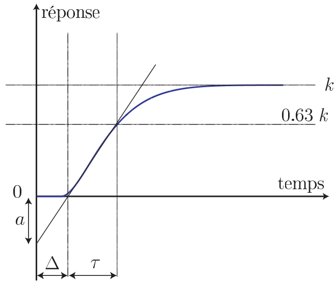
FIGURE 2.18 – Détermination d’un modèle du premier ordre à retard à partir de la réponse à un échelon donné par y(t) = k(1 - e^{-\frac{t-\Delta}{\tau}})\mathbb{I}_{t \geq \Delta} .
