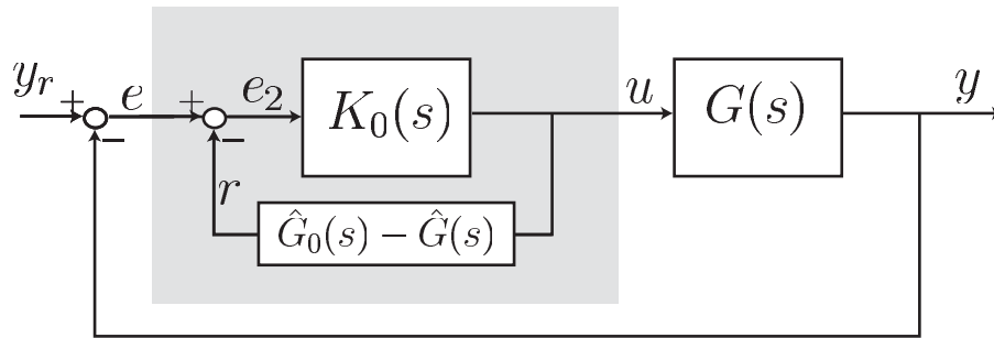
FIGURE 2.19 – Le prédictiveur de Smith (zone grisée).
