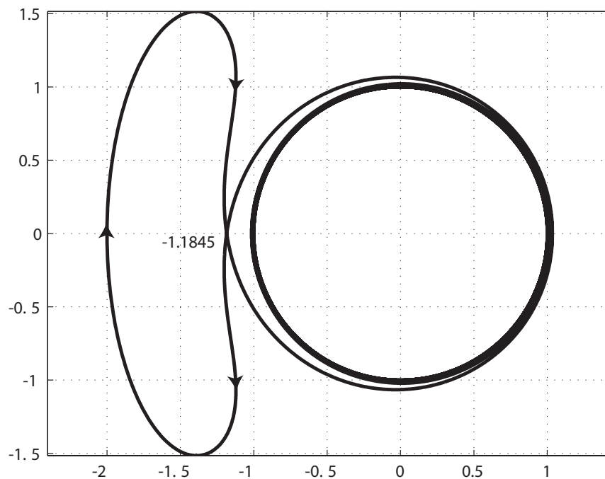
FIGURE 2.10 – Bouclage d'un système à retard.
