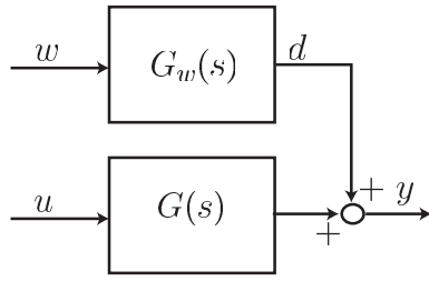
FIGURE 2.4 – Le schéma blocs en boucle ouverte.
