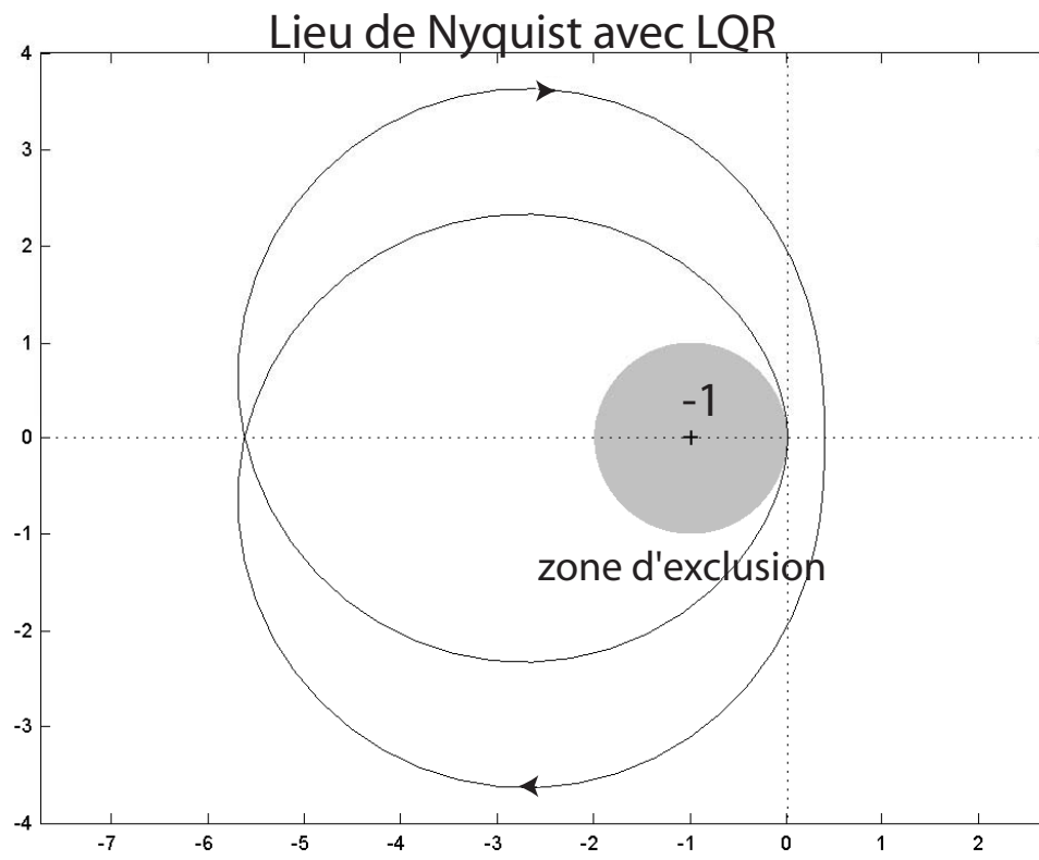
FIGURE 3.12 – Utilisation du LQR en boucle fermée.
