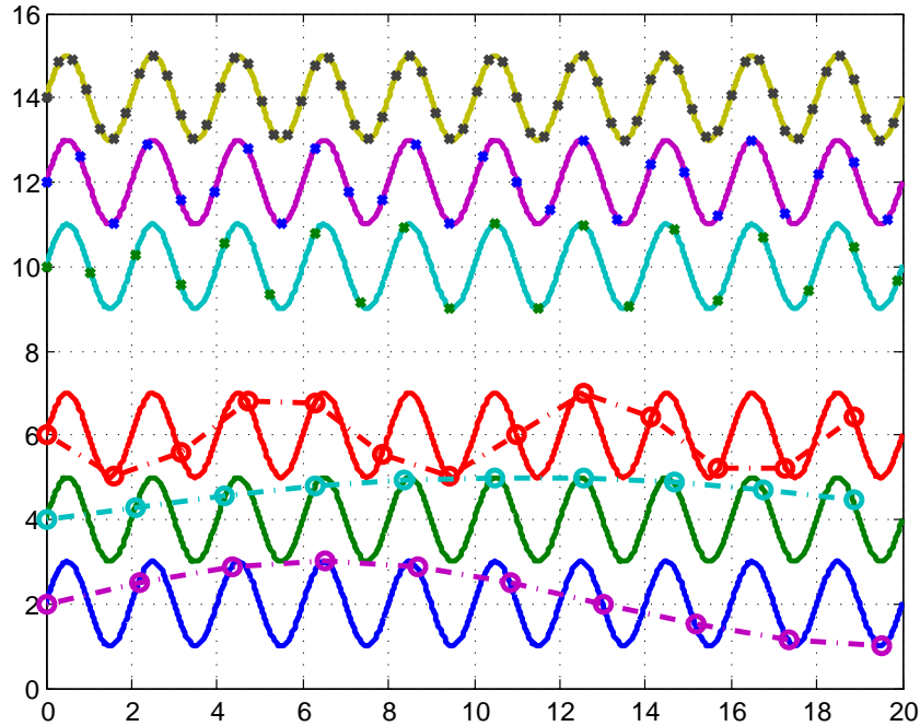
FIGURE D.2 – Apparition du phénomène de repliement spectral lors de l'échantillonnage d'un signal sinusoidal. Des basses fréquences apparaissent lorsque la fréquence d'échantillonnage choisie viole l'hypothèse du Théorème 39 de Shannon (courbes du bas).
