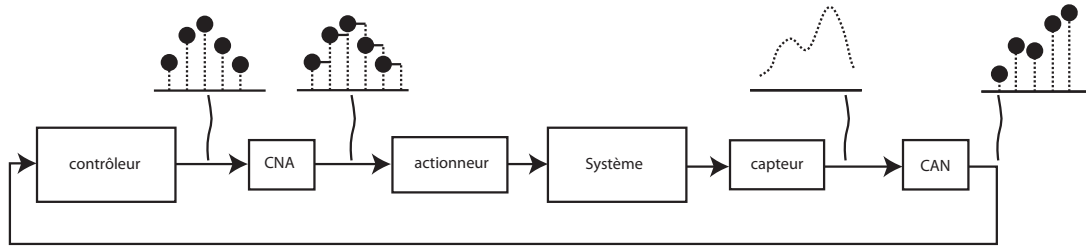
FIGURE D.1 – Schéma d'implémentation numérique d'un algorithme de contrôle.
