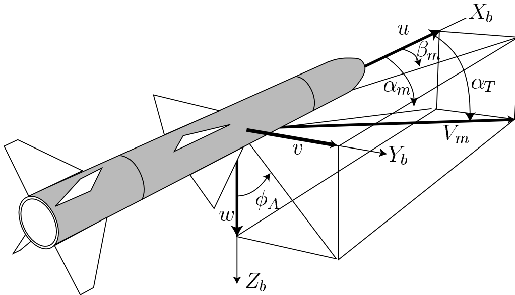
FIGURE 1.1 – Variables décrivant un missile.
