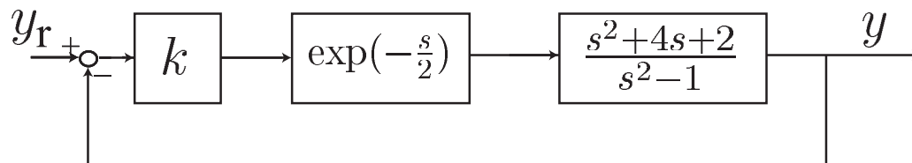
FIGURE 2.10 – Bouclage d'un système à retard.
