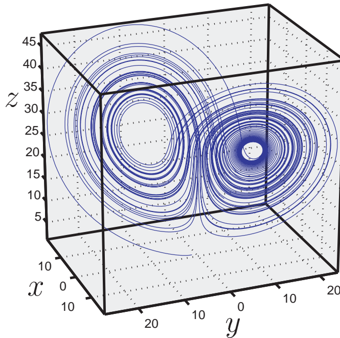
FIGURE 1.12 – Système chaotique de Lorenz.
