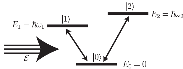
FIGURE 3.2 – Un atome à trois niveaux en interaction avec une lumière laser polarisée linéairement et associée au champ électrique \mathcal{E} \in \mathbb{R} , le contrôle.
